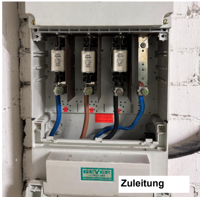
HüP (Hausübergabepunkt), oder HAK (Hausanschlusskasten)
