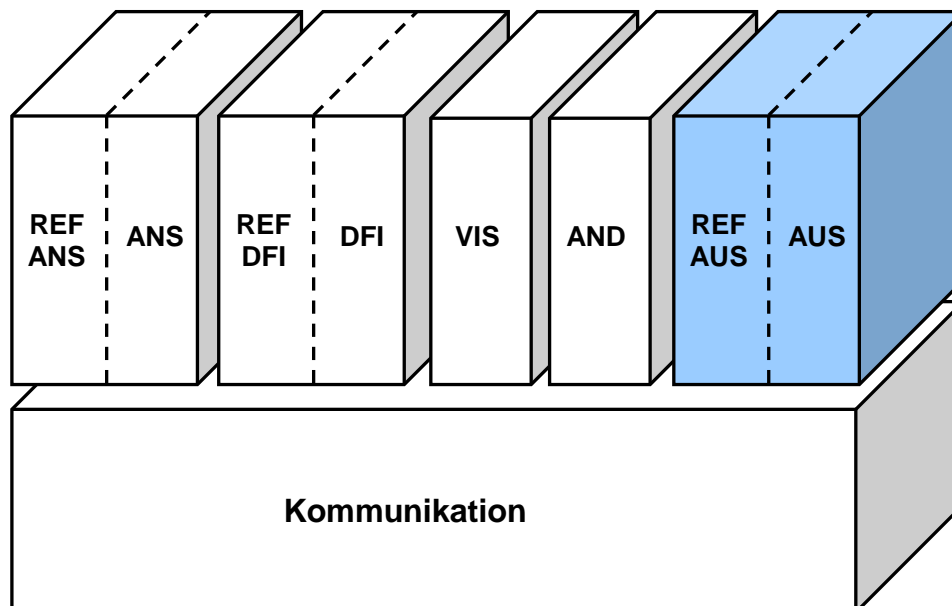
Abbildung 1: Gesamtarchitektur
