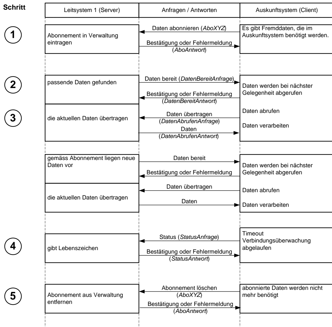
Abbildung 3: Kommunikationsablauf des Abonnementverfahrens
